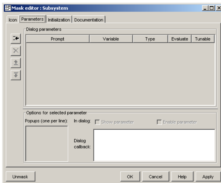
Figure 23 Mask editor -- Parameters tab
